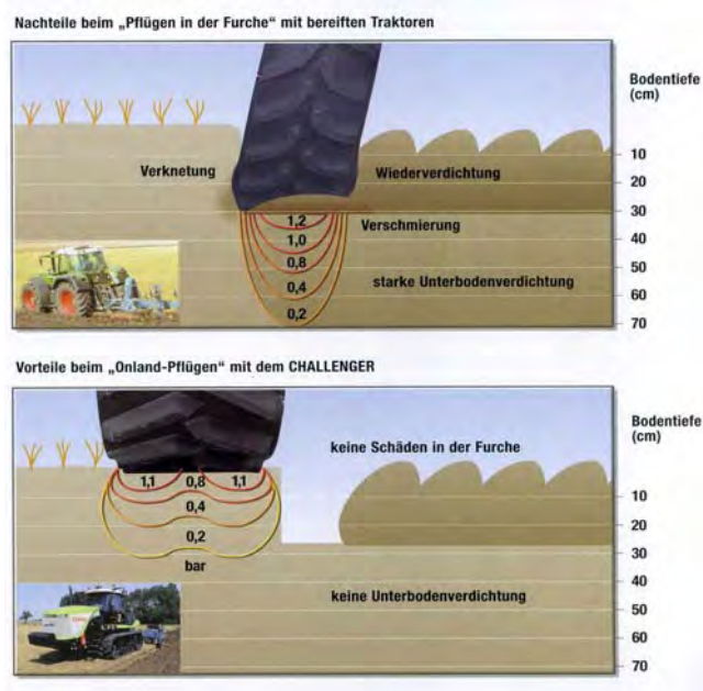
Abbildung 7-13: Negative Auswirkungen konventioneller Pflugarbeit in der Furche und alternative Pflugtechnik (Quelle: Claas o.J., S. 21)
