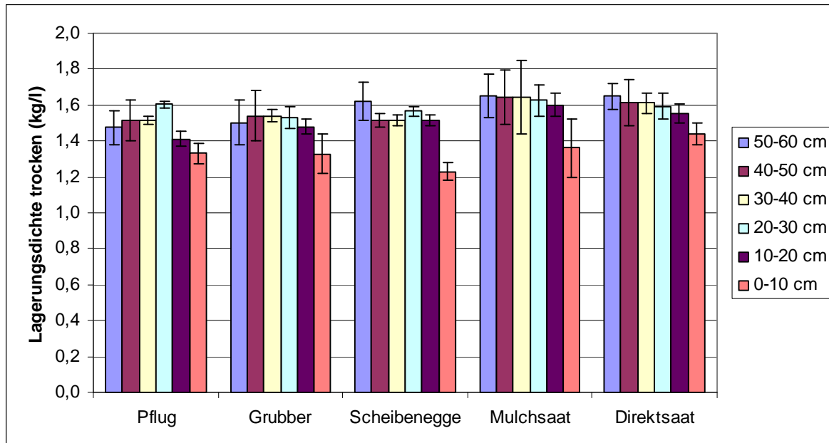
Abbildung 6-1: Lagerungsdichten des Bodens im Frühjahr 2008 auf dem Versuchstandort in Welschbillig in der Eifel in Abhängigkeit von der Bodenbearbeitung und der Tiefe; Mittelwerte von 8 bis 12 Stechringproben ± Standardabweichung (Daten von Bai 2009)
