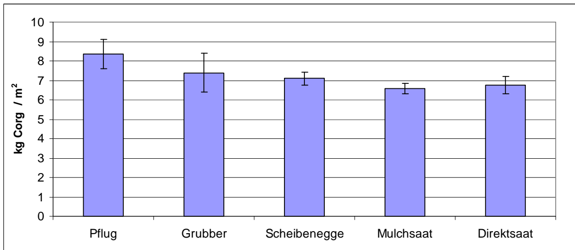
Abbildung 6-5: Organischer Kohlenstoff im Boden bis zur Referenztiefe auf dem Versuchsstandort Dichtelbach/Hunsrück; Mittelwerte von n = 4 Schürfgruben je Variante ± Standardabweichung; die Referenztiefe ist jeweils so tief, dass 812 kg Boden-Trockenmasse pro m 2 berücksichtigt werden; in der Pflugvariante beträgt die Referenztiefe im Mittel genau 60 cm
