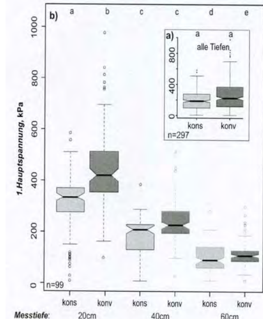
Abbildung 7-14: Mechanische Druckbelastung bei konventioneller und konservierender Bodenbearbeitung (Quelle: Zink 2009, S. 39)
