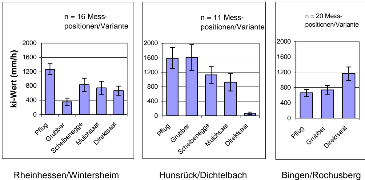
Abbildung 5-3: Infiltrationsleistung in Abhängigkeit von der Bodenbearbeitung auf drei unterschiedlichen Versuchsstandorten in Rheinland-Pfalz; Mittelwerte ± Standardfehler
